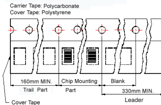
Reel Dimensions
