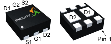
DFN2x2C-6_EP2
