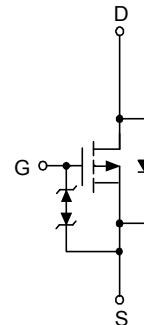
P-Channel MOSFET
