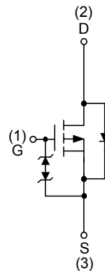
P-Channel MOSFET
