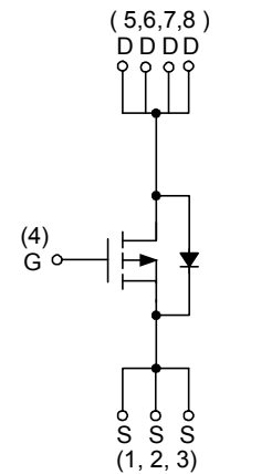
P-Channel MOSFET
