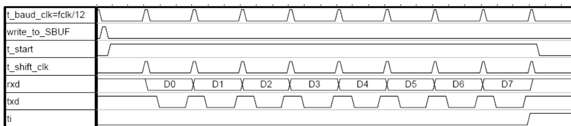
Fig. 8-1: Transmit mode 0
