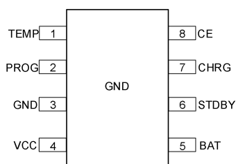
ESOP8
