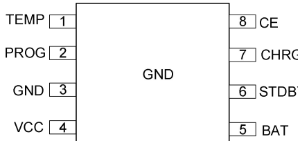
EMSOP8
