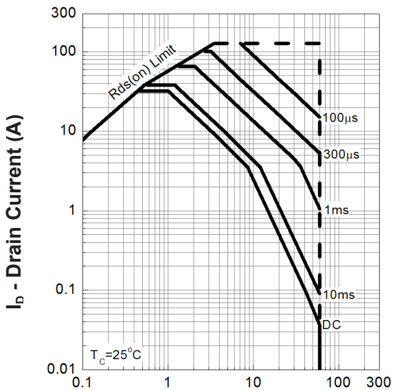
V_{DS} - \text{Drain - Source Voltage (V)}
