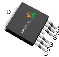
TO-263-6
