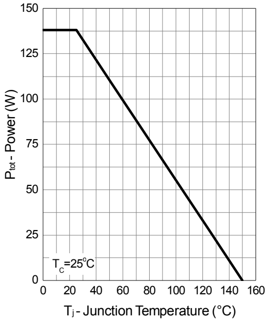
Power Dissipation : TO-220/TO-247
