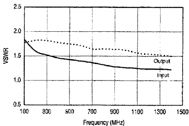
VSWR
