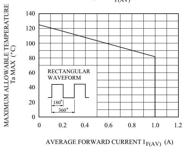
T_a - I_{F(AV)}
