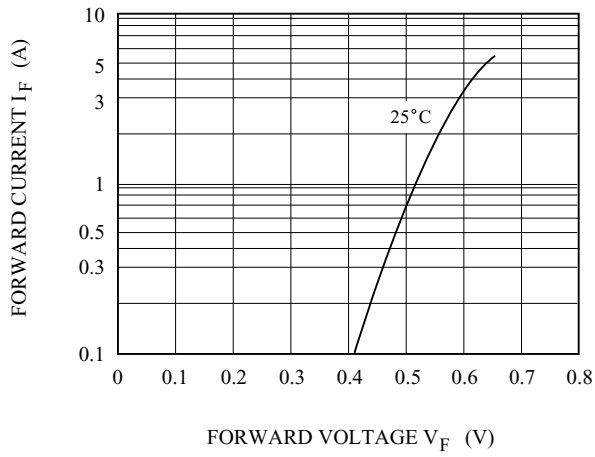
I_F - V_F
