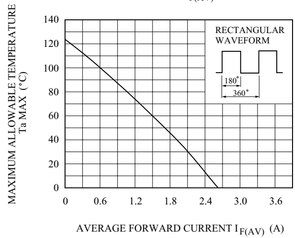
T_a - I_{F(AV)}
