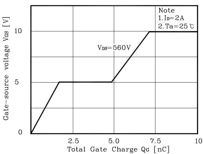
Fig. 6 V_{GS} - Q_G
