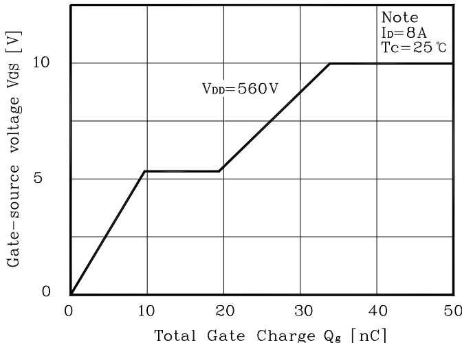
Fig. 6 V_{GS} - Q_g
