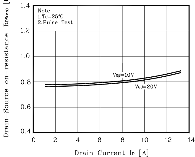
Fig. 3 R_{DS(on)} - I_D
