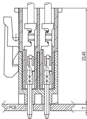
PCB ASS'Y
