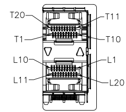
DETAIL A 1:1
