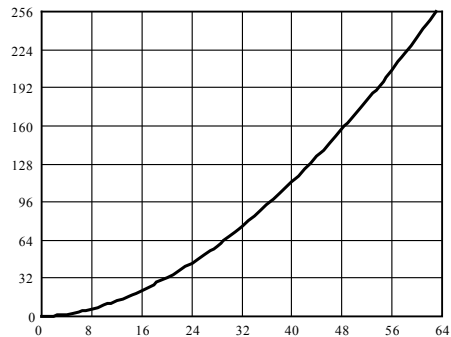
图7 伽玛补偿修正曲线 (64 级)
