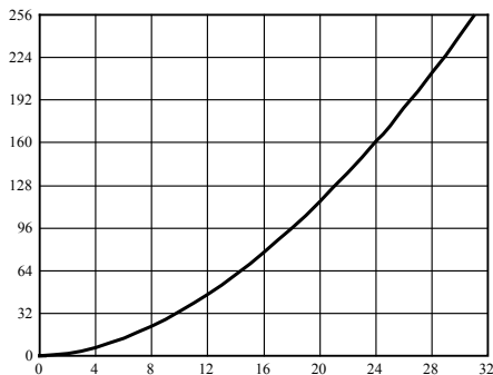
图6 伽玛补偿修正曲线 (32 级)
