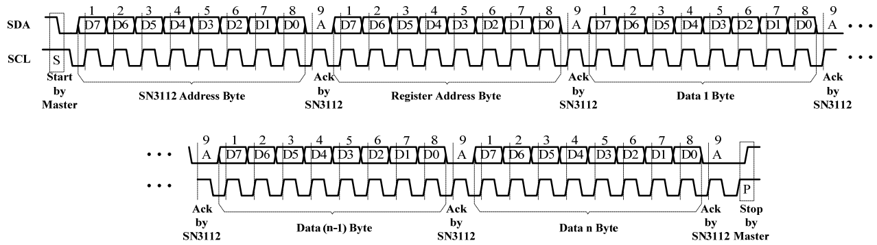
图5 地址自加方式写入 SN3112-09
