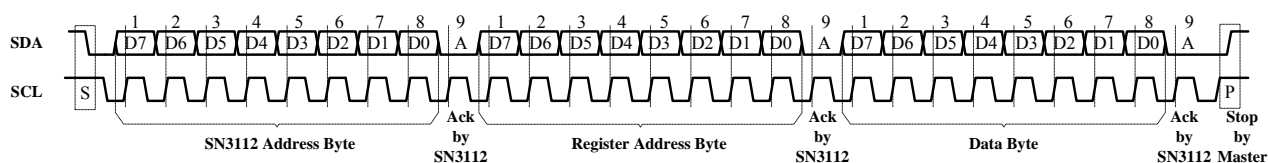
图 4 典型方式写入 SN3112-09
