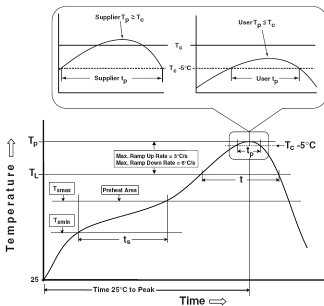
图8 回流焊接温度曲线
