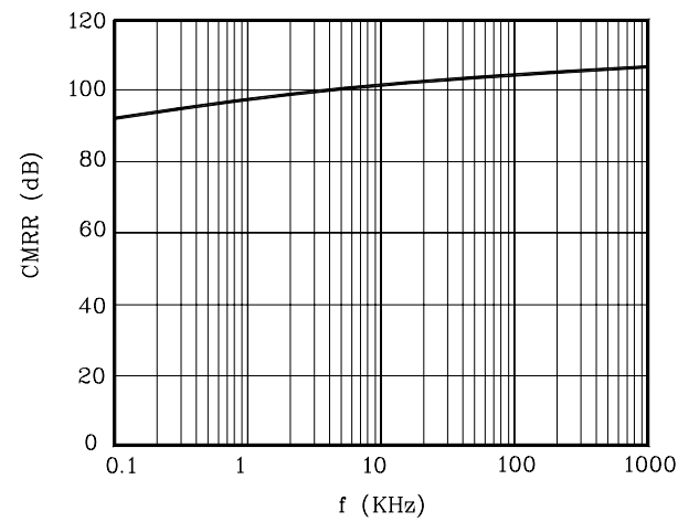
Fig. 5 CMRR-f
