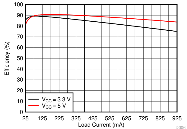
SN6505A-Q1 + Würth 750315240
