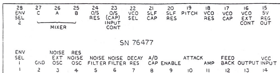
IC Pinout
