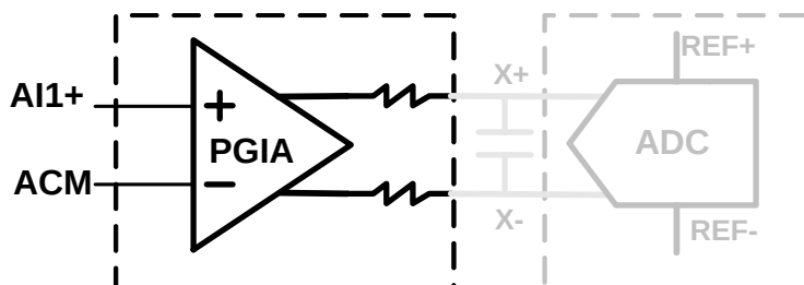
AMPCHS[2:0]="0110"
