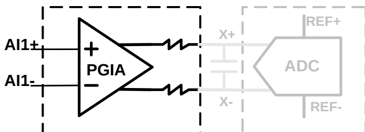
AMPCHS[3:0]="0011"
