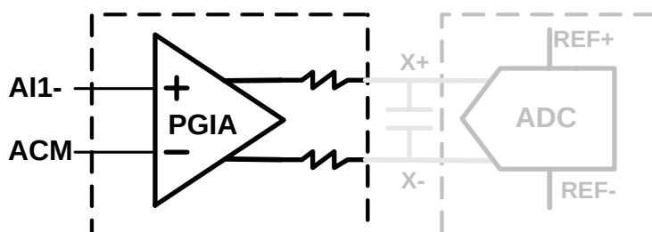
AMPCHS[3:0]="0011"
