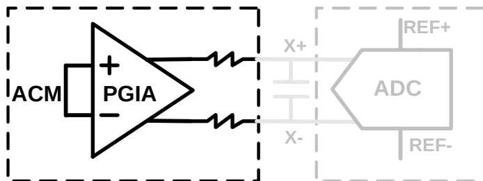
AMPCHS[2:0]="0110"
