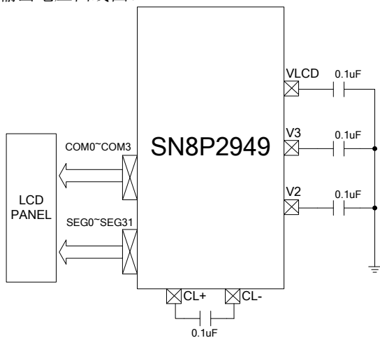
1/3 偏压, C 型 LCD 应用电路
