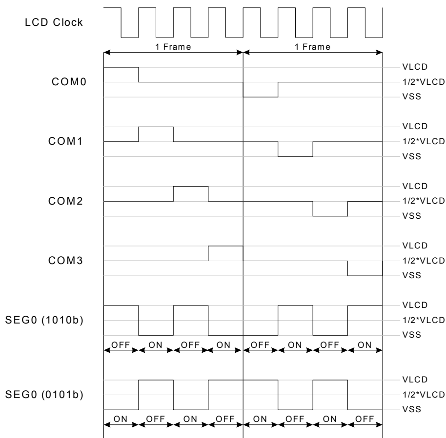
LCD 驱动波形，1/4 duty, 1/2 bias
