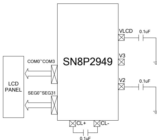
• 1 1/2 偏压, C 型 LCD 应用电路
