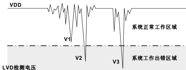
掉电复位电路图
