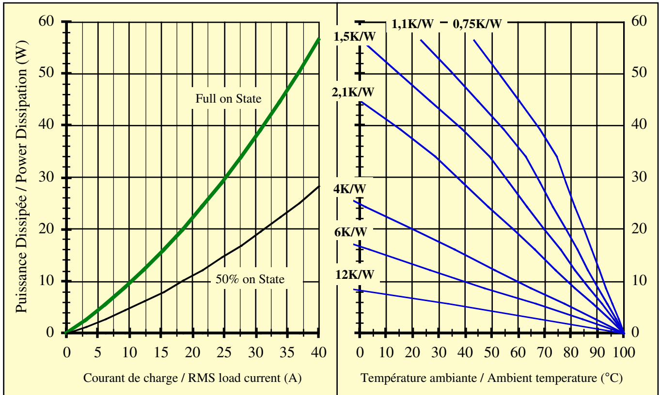
Fig. 2 Courbes thermiques &amp; Choix dissipateur thermique / Thermal curves and heatsink choice
