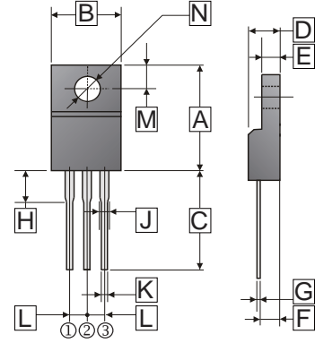
ITO-220
