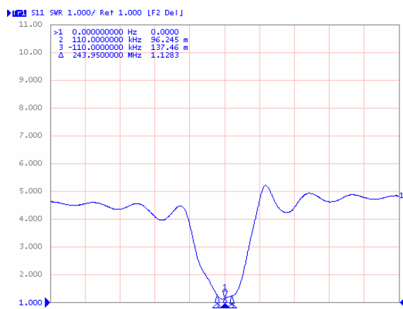
VSWR S11
