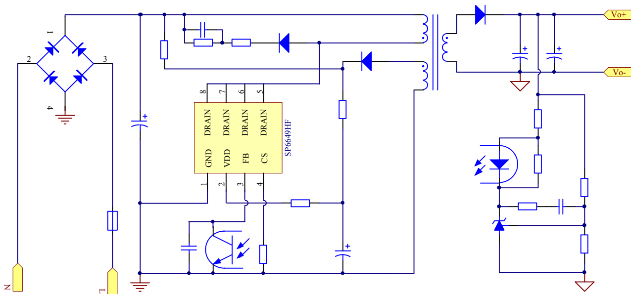
应用 1.适配器方案
