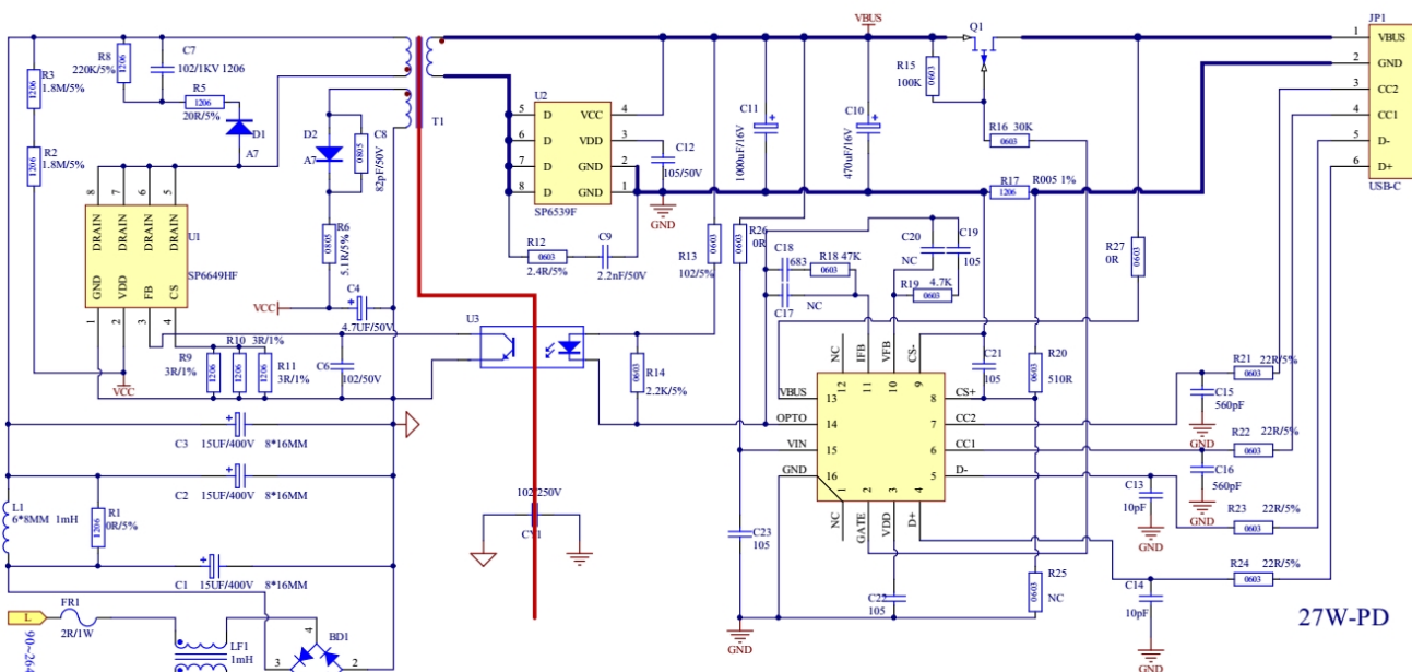
应用 2.充电器方案
