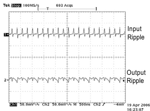
Ripple 2X Flash 1000mA, V_{IN}=3.6V
