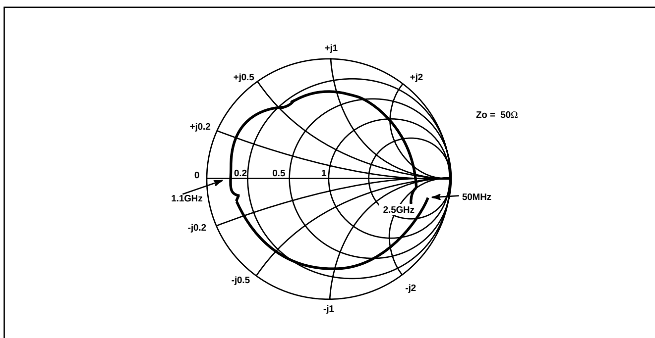
Fig. 4 R.F. input impedance
