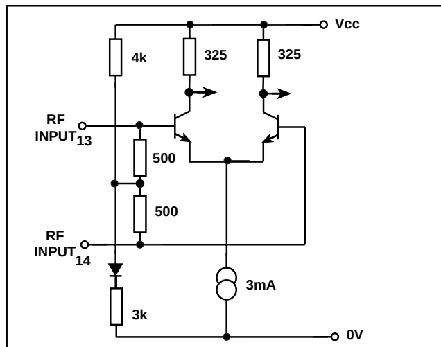
Fig. 7b RF inputs
