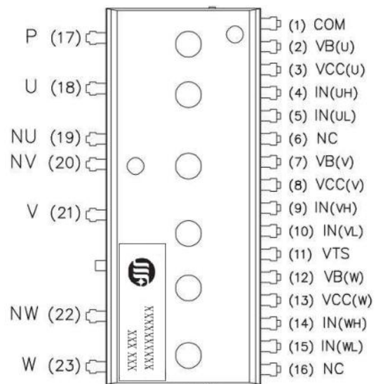
图 2：模块引脚分布示意图
