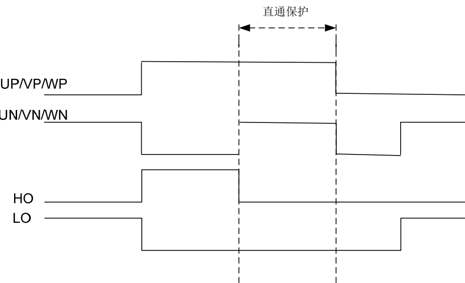
图 9：直通保护
