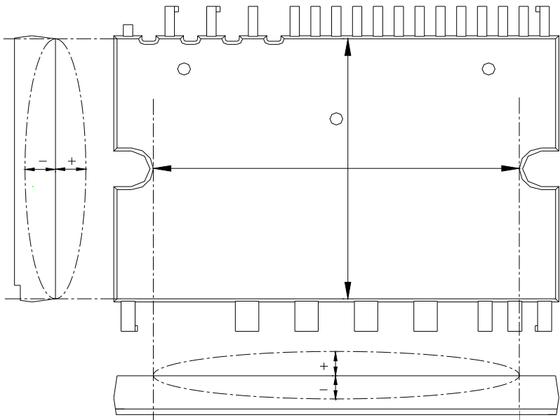
图 6：平面度检测位置
