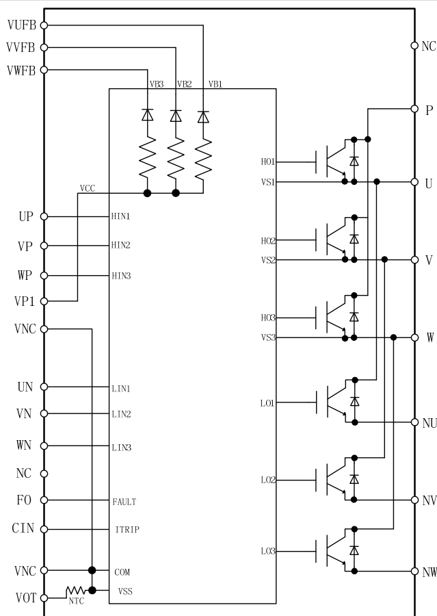
图 1: 内部电路图
