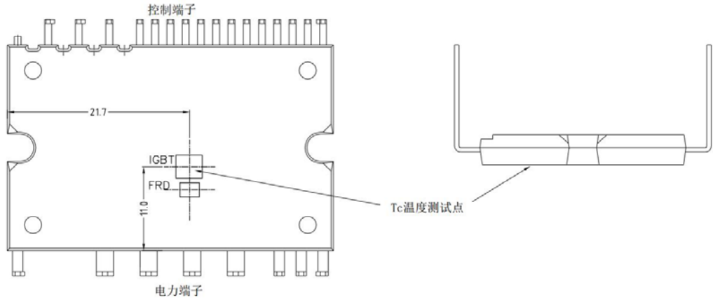
图 3: 壳温测试点
