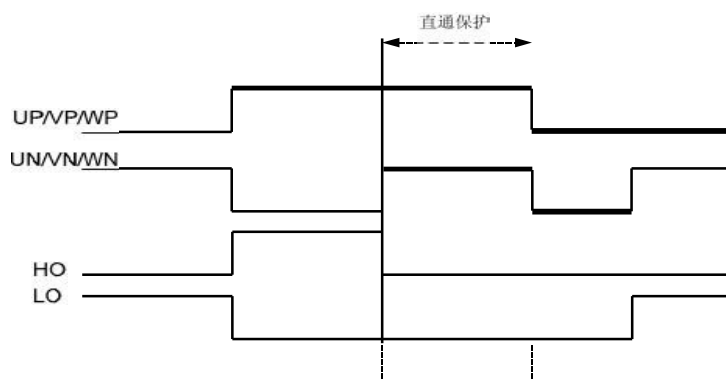
图 10: 直通保护
