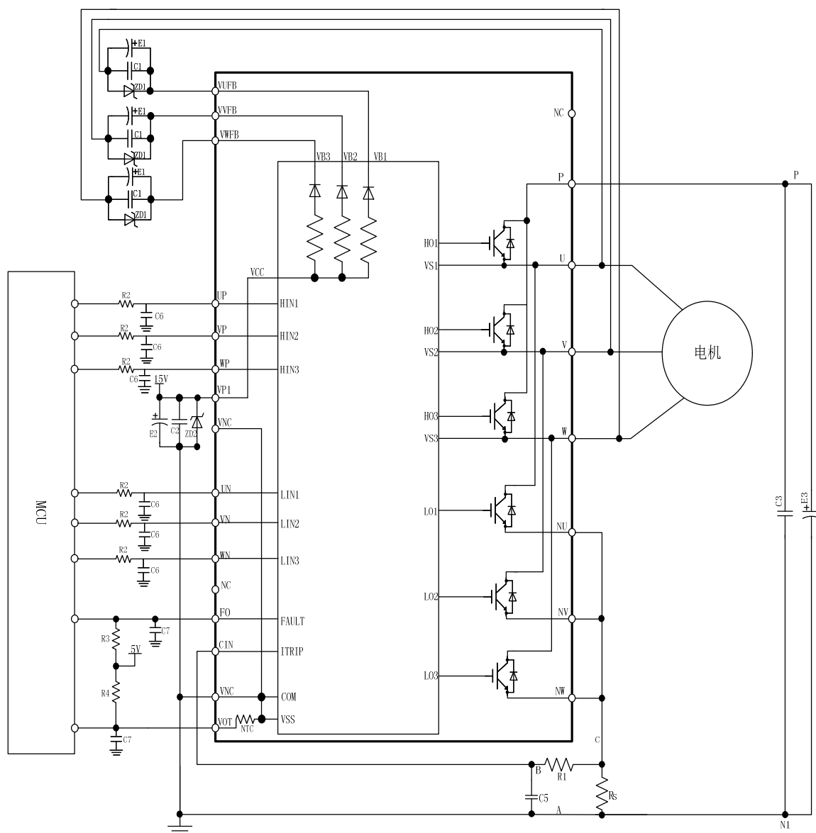
图 16: 典型应用电路
