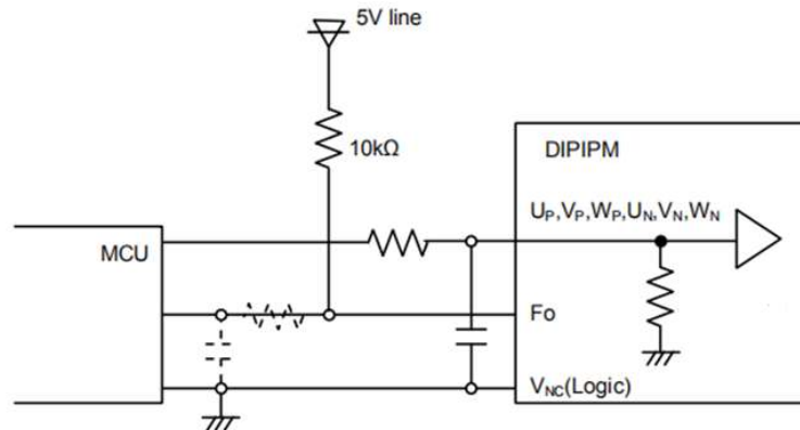
图 14: 推荐的 MCU 输入输出接口电路
