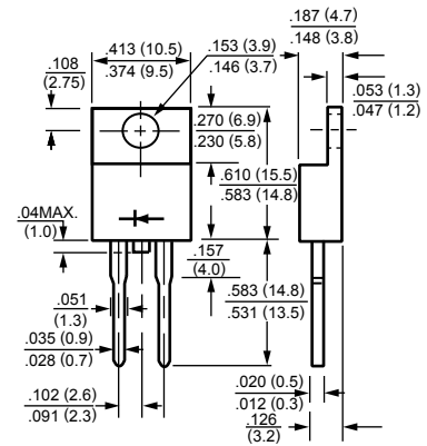
TO-220A
