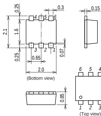
外形図 1323
