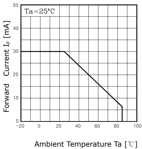
Fig. 3 I_F - T_a
