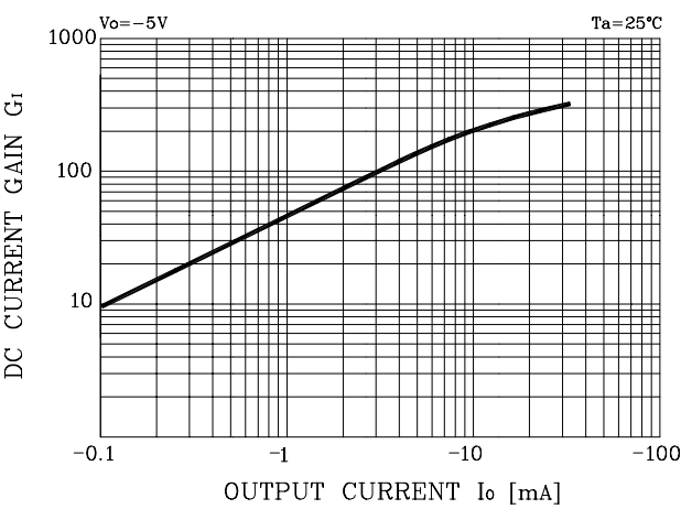
Fig. 3 G_I - I_o
