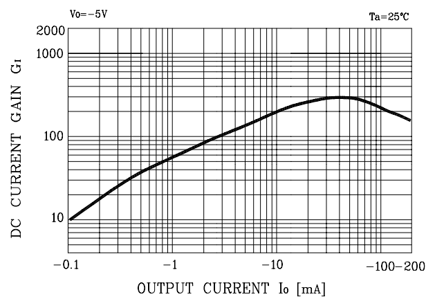
Fig. 3 G_I - I_O
