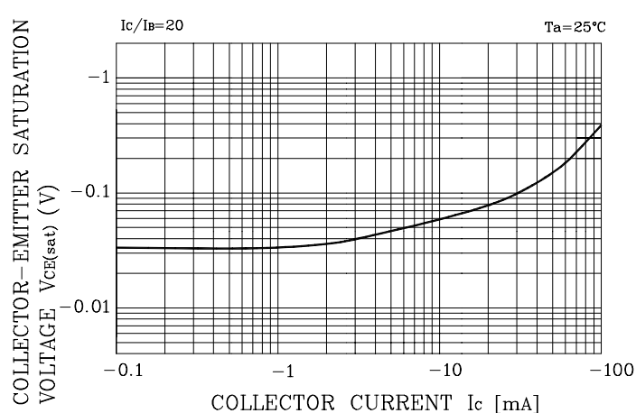
Fig. 2 V_{CE(SAT)} - I_C
