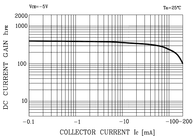
Fig. 1 h_{FE} - I_C
