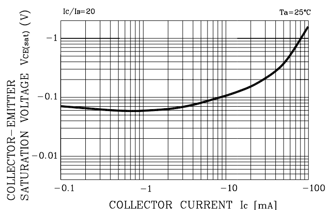
Fig. 2 V_{CE(SAT)} - I_C
