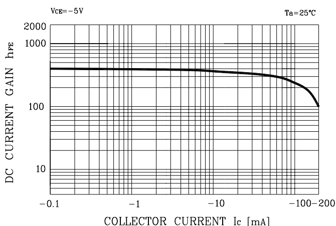
Fig. 1 h_{FE} - I_C
