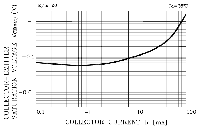
Fig. 2 V_{CE(SAT)} - I_C
