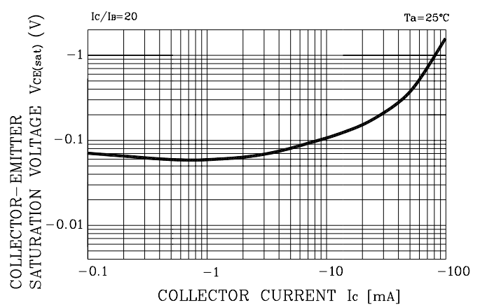
Fig. 2 V_{CE(SAT)} - I_C
