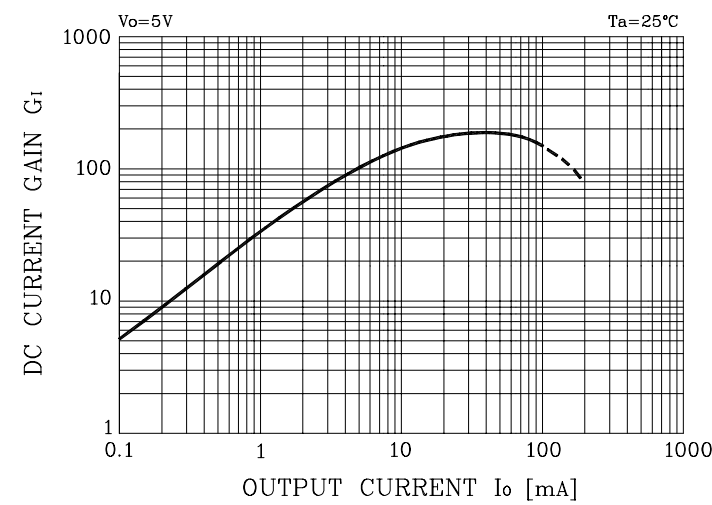
Fig. 3 G_I - I_O
