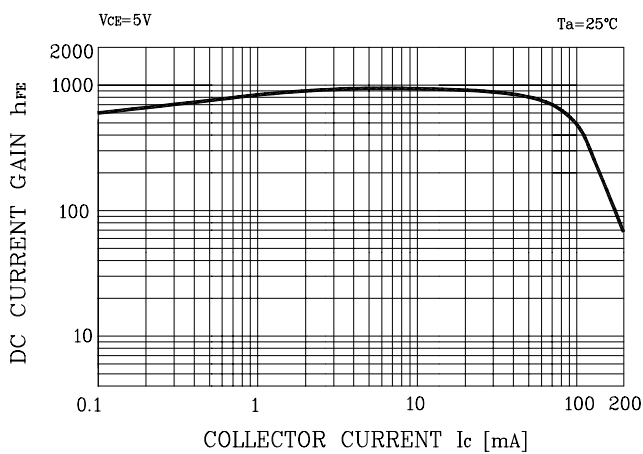
Fig. 1 h_{FE} - I_C
