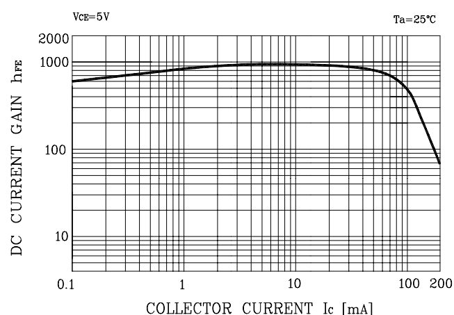
Fig. 1 h_{FE} - I_C
