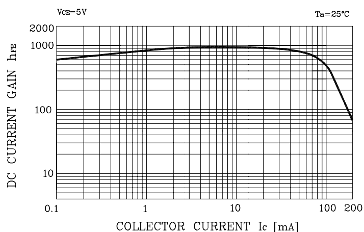
Fig. 1 h_{FE} - I_C
