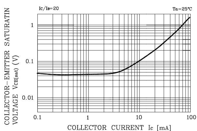
Fig. 2 V_{CE(SAT)} - I_C
