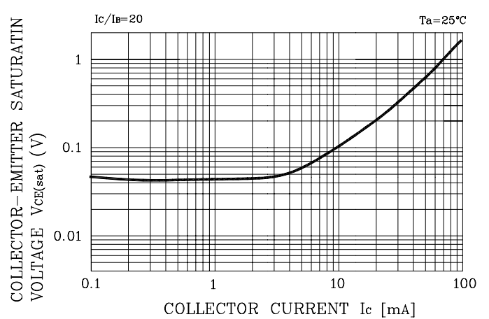
Fig. 2 V_{CE(SAT)} - I_C
